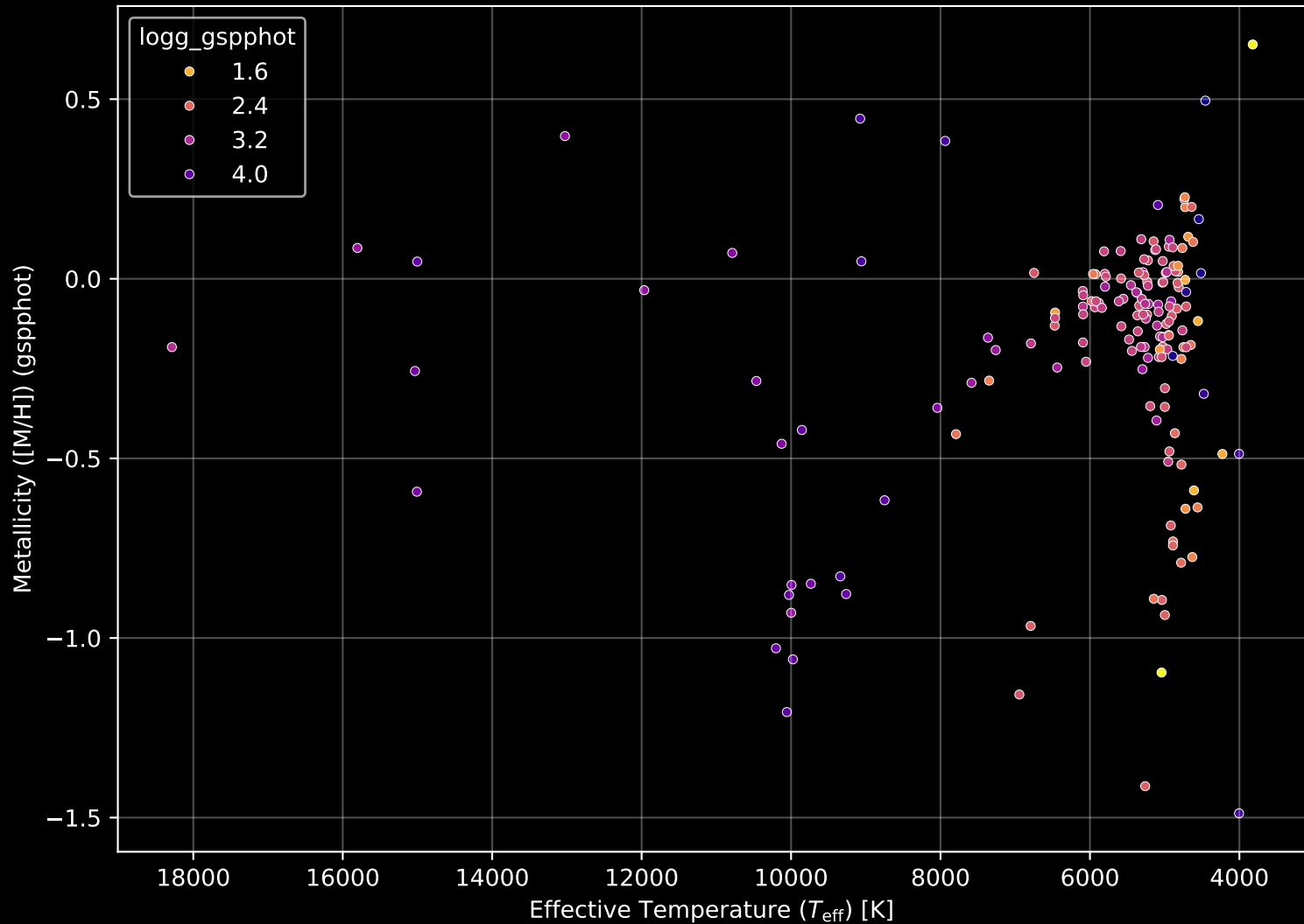
APOGEE DR17 Field: [235+00] Stellar Population Parameters (n= 170)
